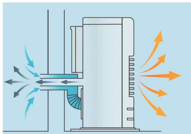
Las estufas a tiro forzado aseguran ambientes más saludables al interior del hogar. El oxígeno necesario para la combustión es tomado desde el exterior gracias a un pequeño ducto de 8cm, que a su vez expulsa las emisiones hacia afuera.
